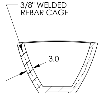
SECTION A-A SCALE 1 : 20
