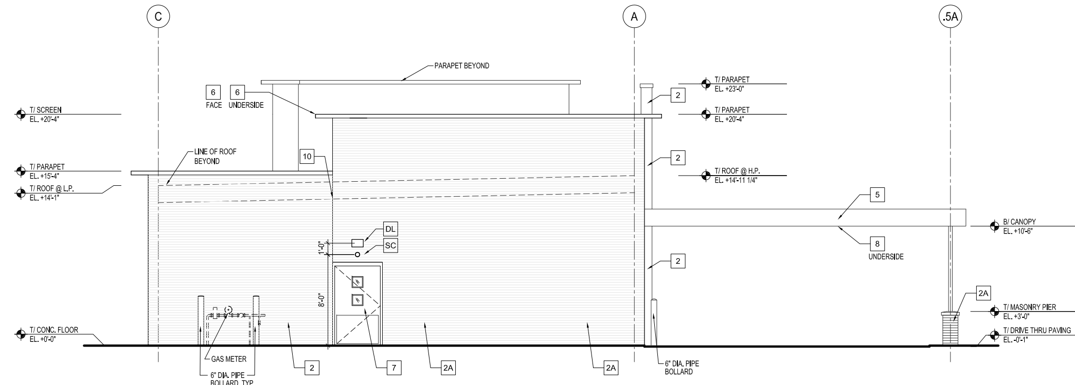
REAR - NORTH ELEVATION Scale: N.T.S.
