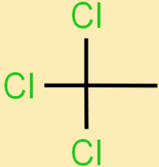
1,1,1- Trichloroethane
