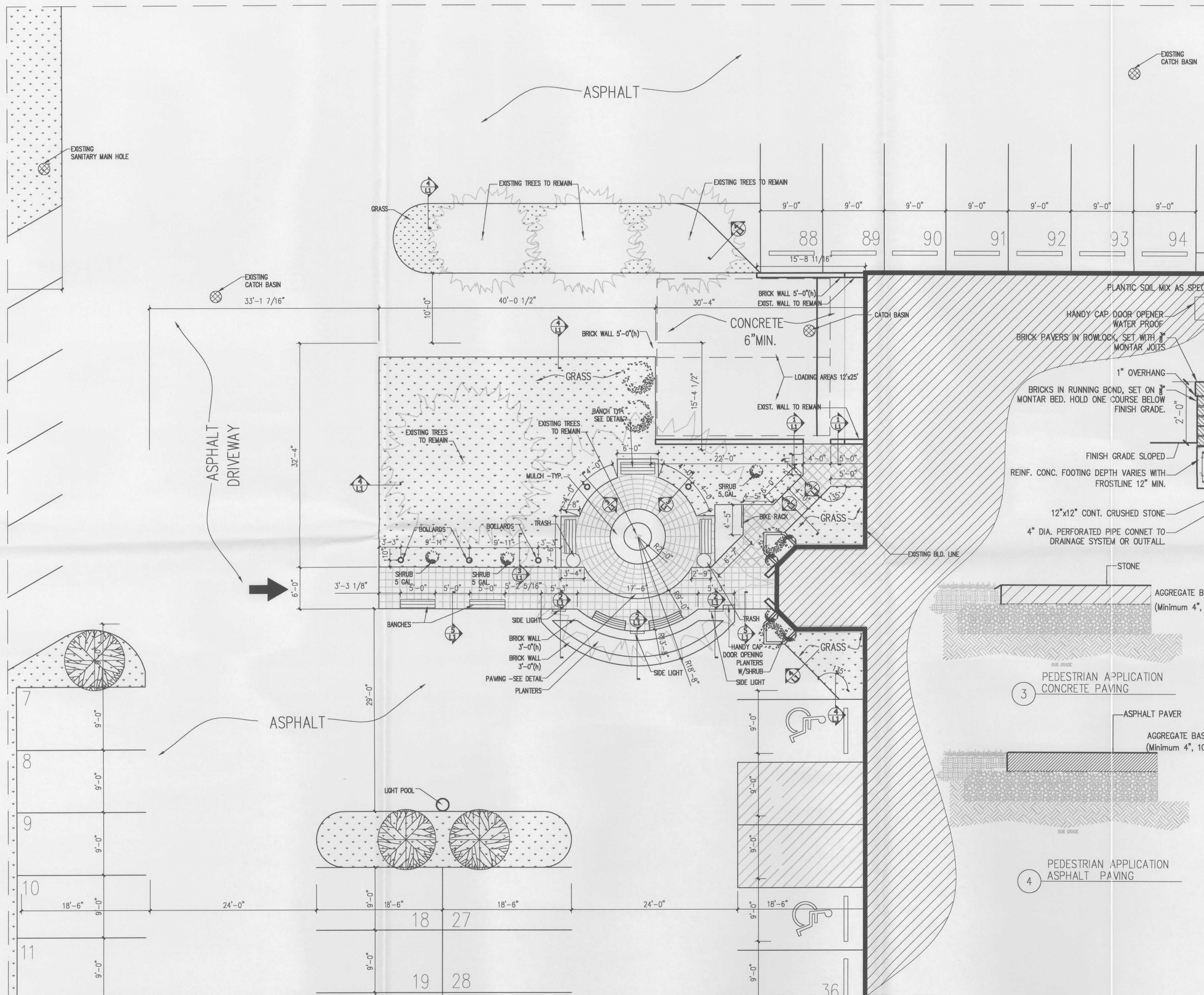
1 PLAN Scale: 1/8"=1'-0"
