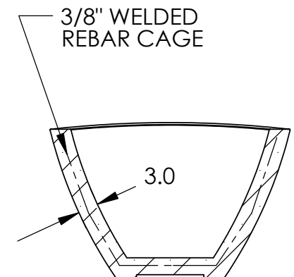
SECTION A-A SCALE 1 : 20
