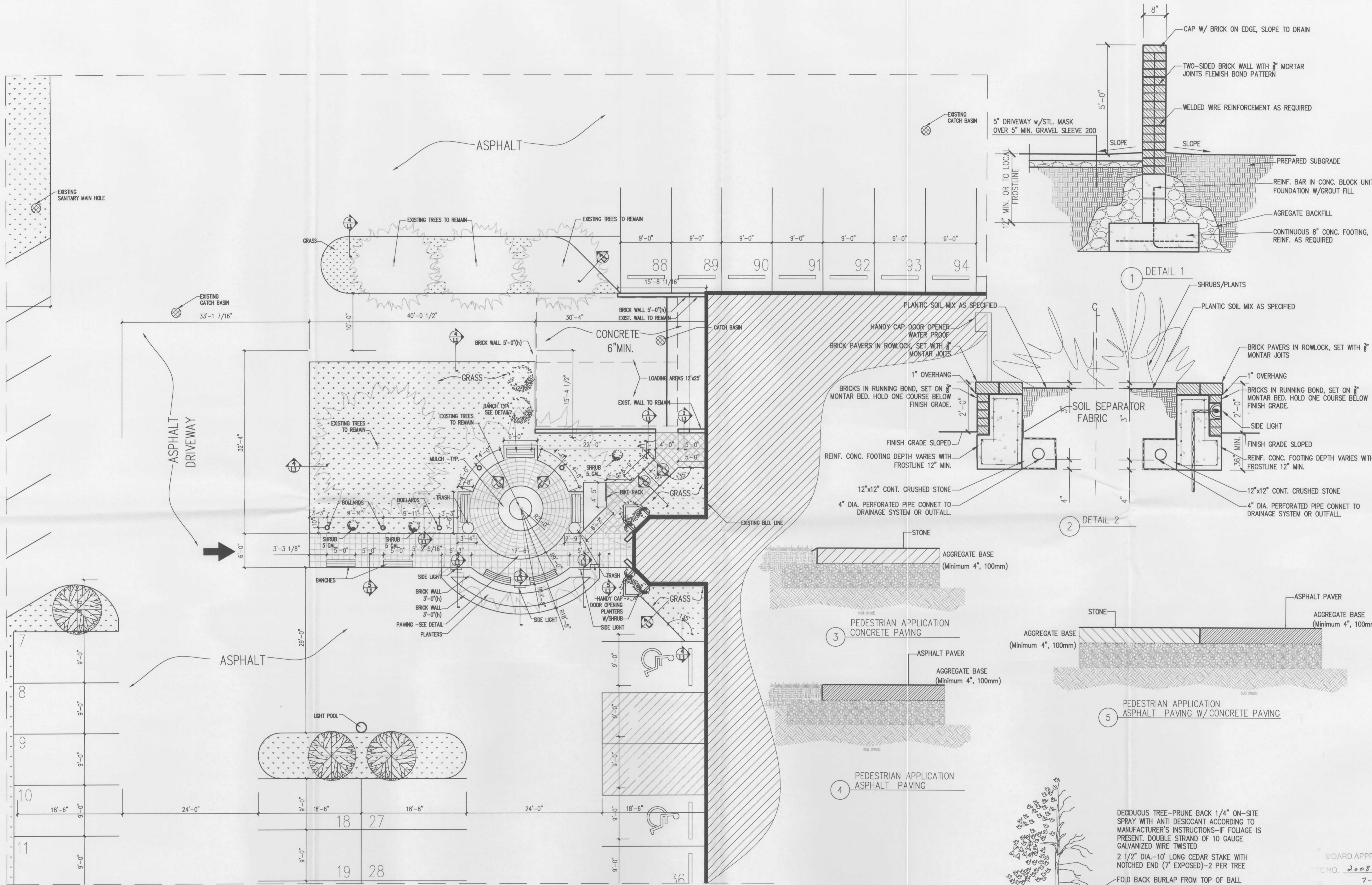
1 PLAN Scale: 1/8"=1'-0"
